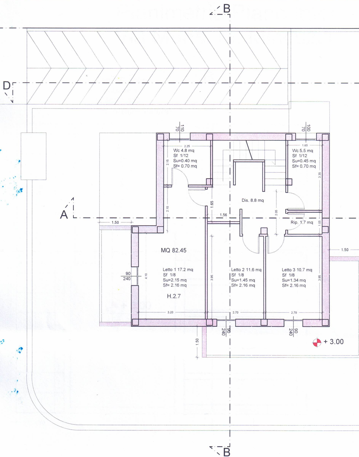
Planimetria Piano Primo
